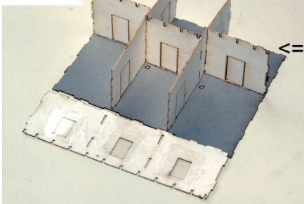
4. => „Loch außen“
