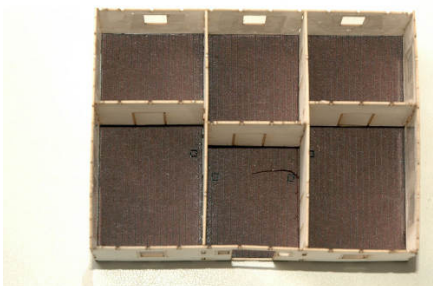
7. Böden einkleben
